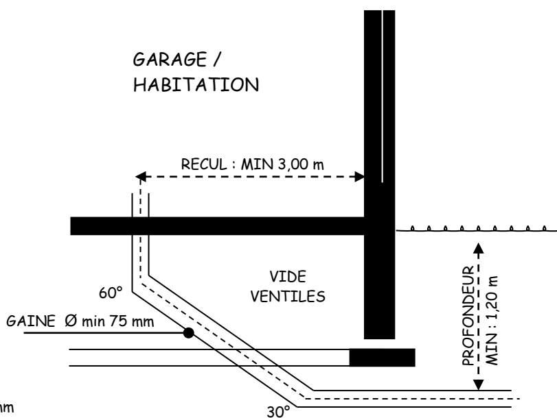
DETAIL 2 : coupe transversale
