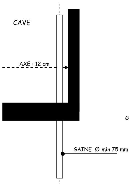
DETAIL 1 : coupe longitudinale
